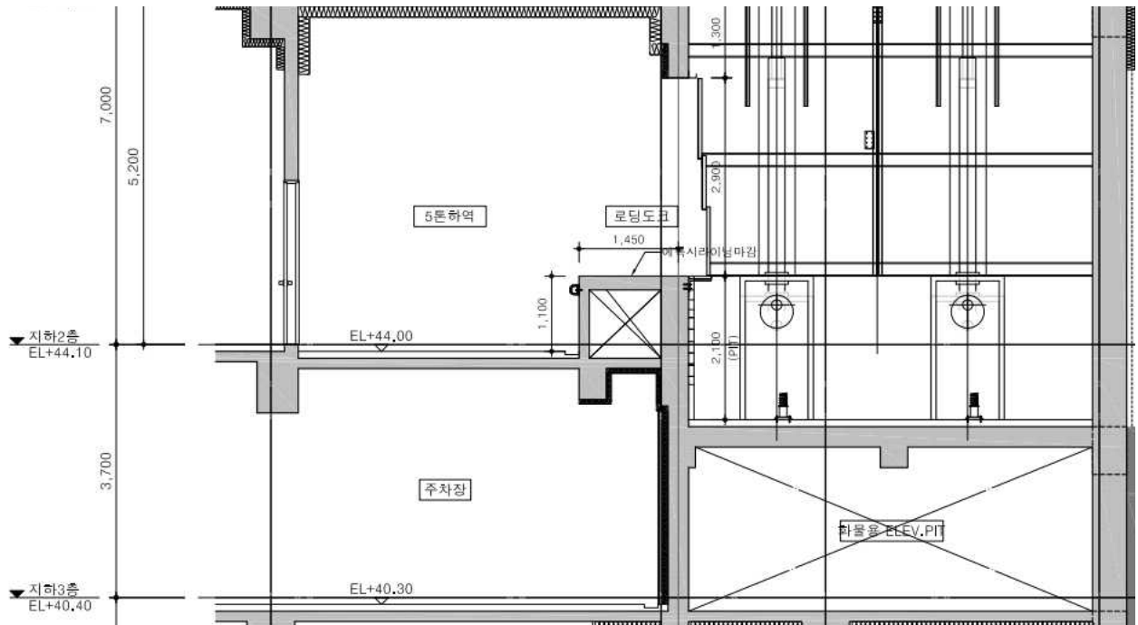
장치 반입구 단면도
