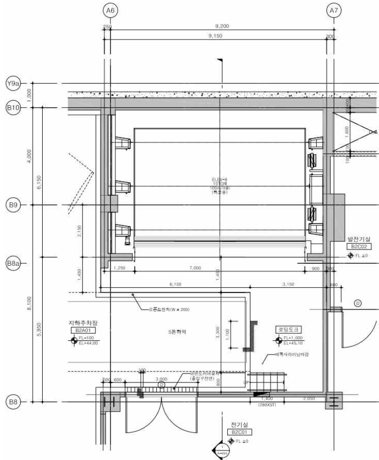
장치 반입구 평면도
